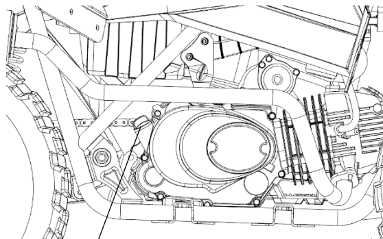
Vareta do óleo
